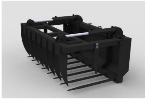
Вилы челюстные
